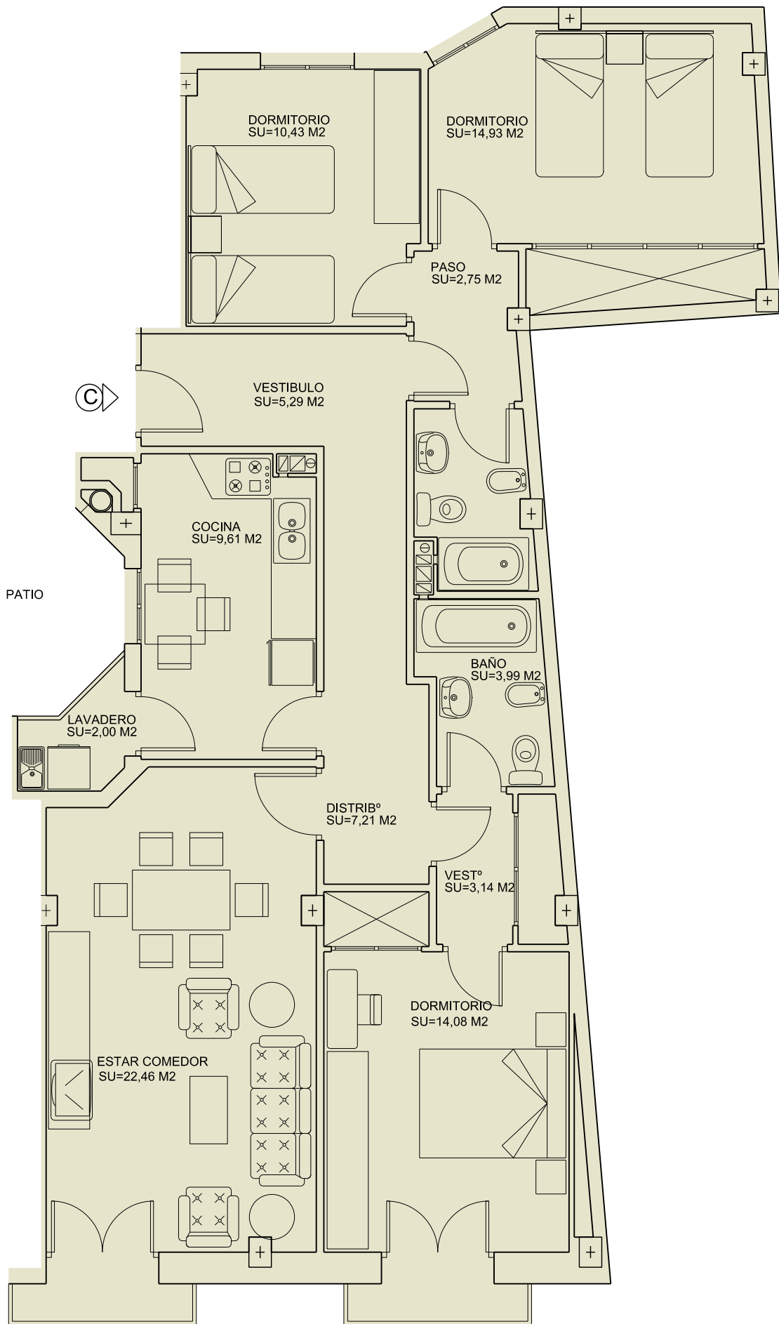
CUADRO DE SUPERFICIES DE PLANTA PRIMERA
